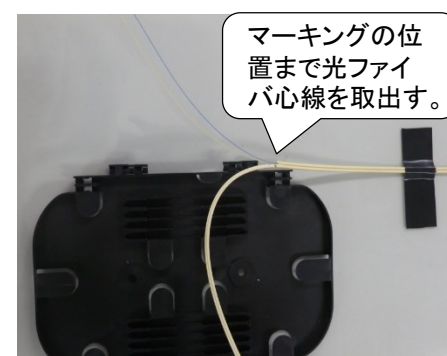
—H.光ファイバ心線の取出し(3)—
