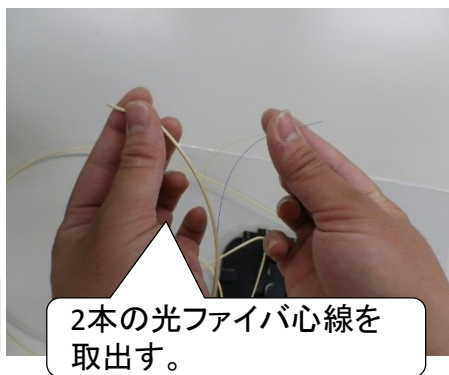
—F.光ファイバ心線の取出し(1)—
