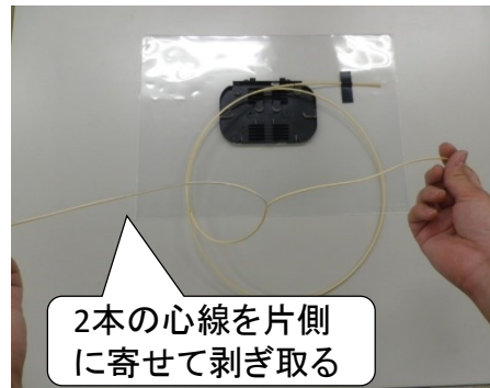
—C.外被の剥ぎ取り1—
