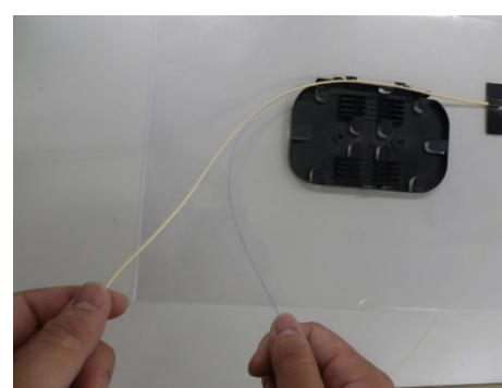
—F.光ファイバ心線の取出し(2)—
