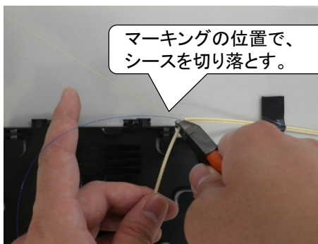
—I.ケーブルシースの切り落し—
