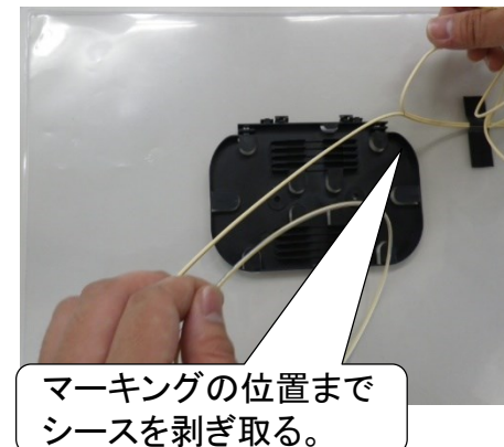
—H.光ファイバ心線の取出し(3)—
