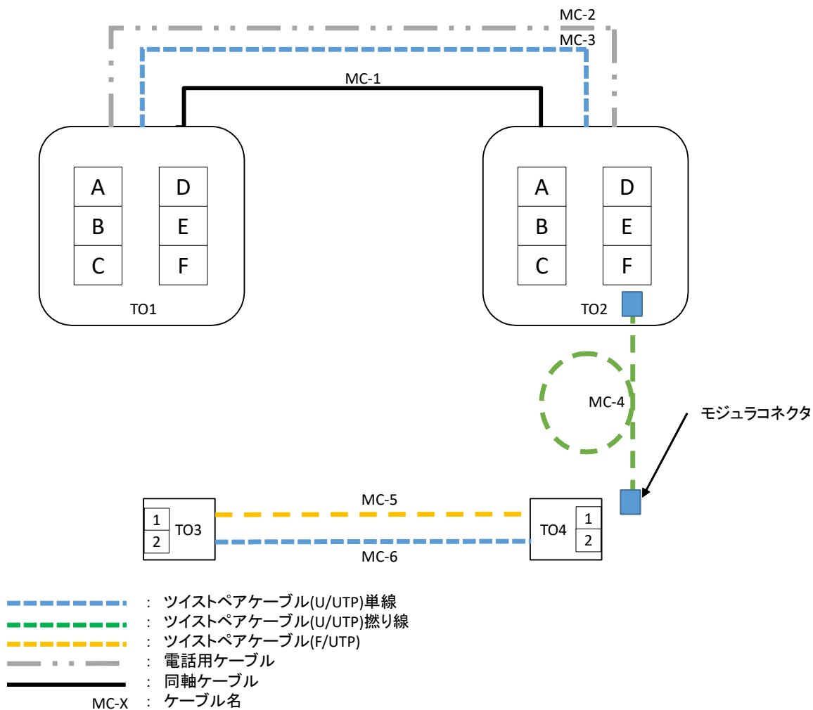
図4 配置図
