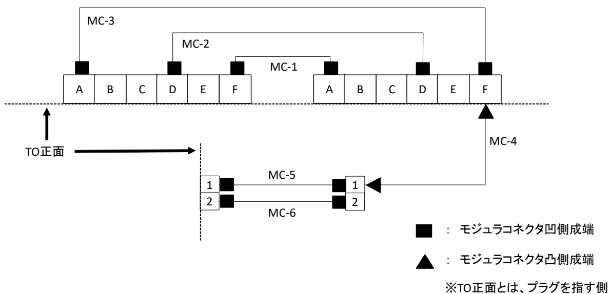
図5 配線図
