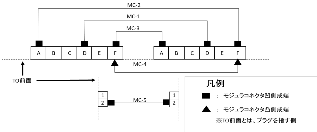
図4 配線図
