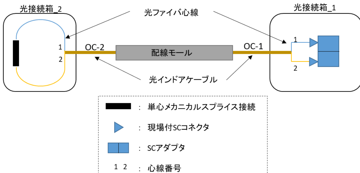
図2 光ファイバ心線接続図
