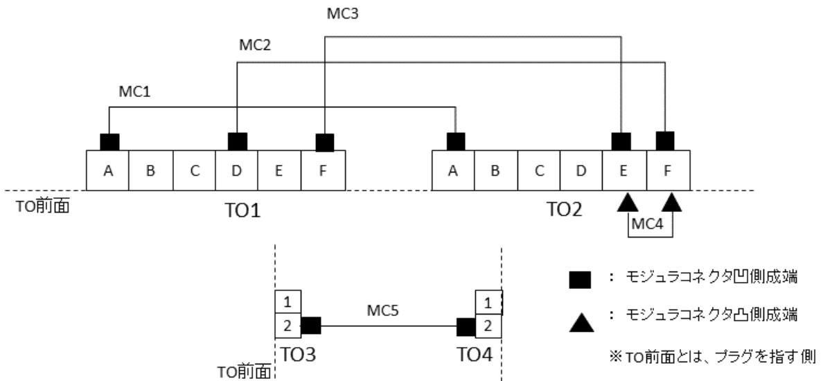
図4 配線図
