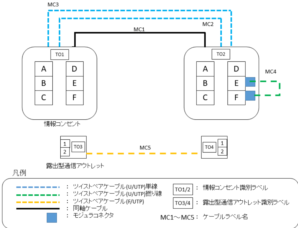
図3 配置図
